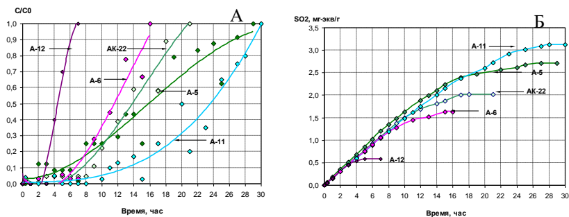
Рисунок 2 – Кривые проскока (А) и сорбции (Б) диоксида серы на волокнистых анионитах ФИБАН при относительной влажности воздуха, обеспечивающей достижение эффективного коэффициента влагоемкости K^0 = 2 : АК-22 – 54%, А-5 – 36%, А-6 – 30%, А-11 – 40%, А-12 – 30%.
