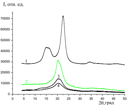
Рисунок 4 – Дифрактограммы хлопковой целлюлозы (а), древесной сульфитной целлюлозы (1), катионной хлопковой целлюлозы CЗ_{кат.} = 0,24 (2), катионных древесных целлюлоз: CЗ_{кат.} = 0,11 (3), CЗ_{кат.} = 0,33 (4)
