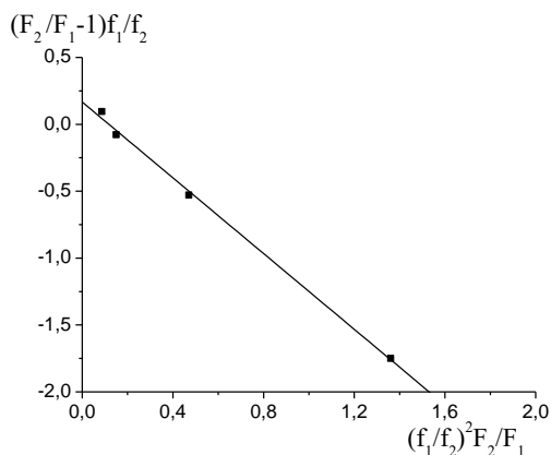
Рисунок 1 – Определение констант сополимеризации МАА и АМПСNa методом Файнмана-Росса
