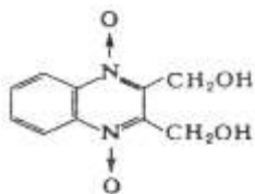
Рисунок 1. Структурная формула диоксидина
