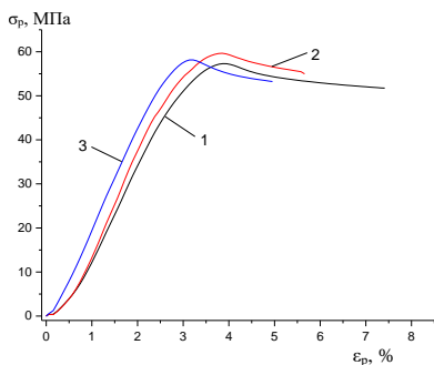
Рисунок. Диаграммы растяжения пленок поли-L-лактида
