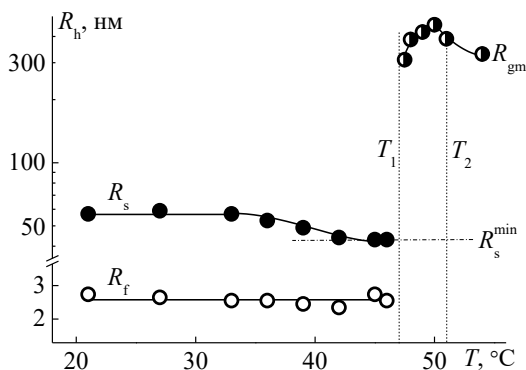
Рис. 3. Температурные зависимости R_f и R_s для раствора К8А-(ПОПК-блок-ПИПО) при концентрации c = 0.0050 г/см 3 и \text{pH} = 5.0 .
