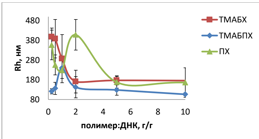
Рис. 2. Зависимость гидродинамического радиуса полиплексов от массового соотношения полимер:ДНК (фосфатный буферный раствор, pH 7.4).
