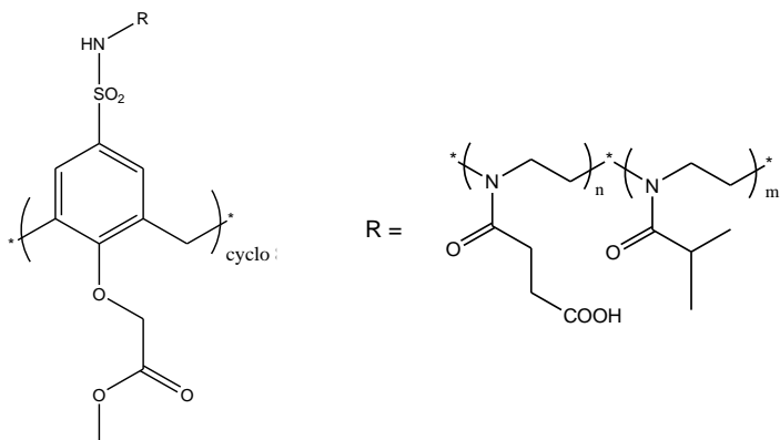
Рис. 1. Структура К8А-(ПОПК-блок-ПИПО).
