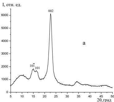
Рисунок 4 – Дифрактограммы хлопковой целлюлозы (а), древесной сульфитной целлюлозы (1), катионной хлопковой целлюлозы CЗ_{кат.} = 0,24 (2), катионных древесных целлюлоз: CЗ_{кат.} = 0,11 (3), CЗ_{кат.} = 0,33 (4)
